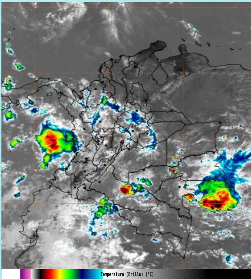
Imagen GOES 19 East Canal Infrarrojo, 23 de septiembre de 2026 - Hora 11:40 HLC. Fuente: https://bart.ideam.gov.co GOES 19
